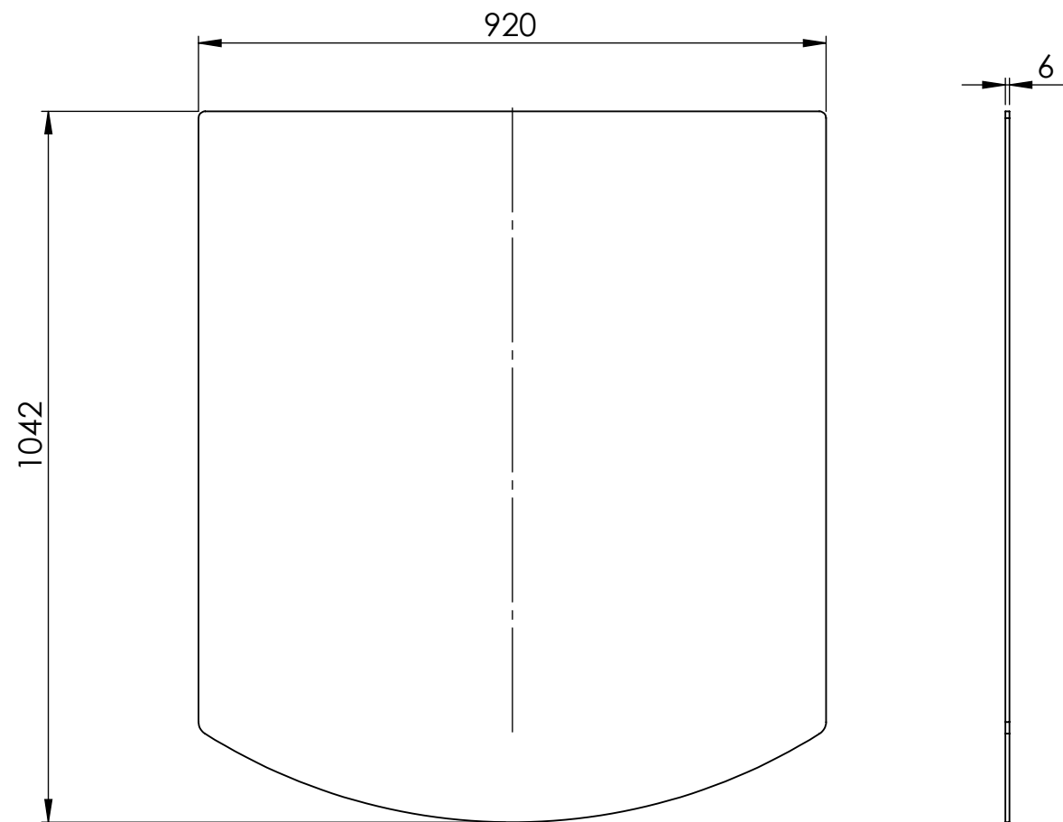
Universal (3535-0102)
