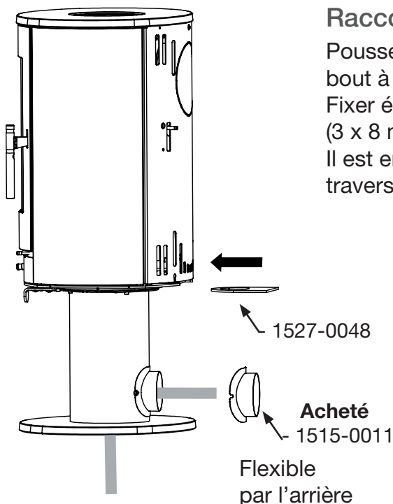
Flexible par le sol
